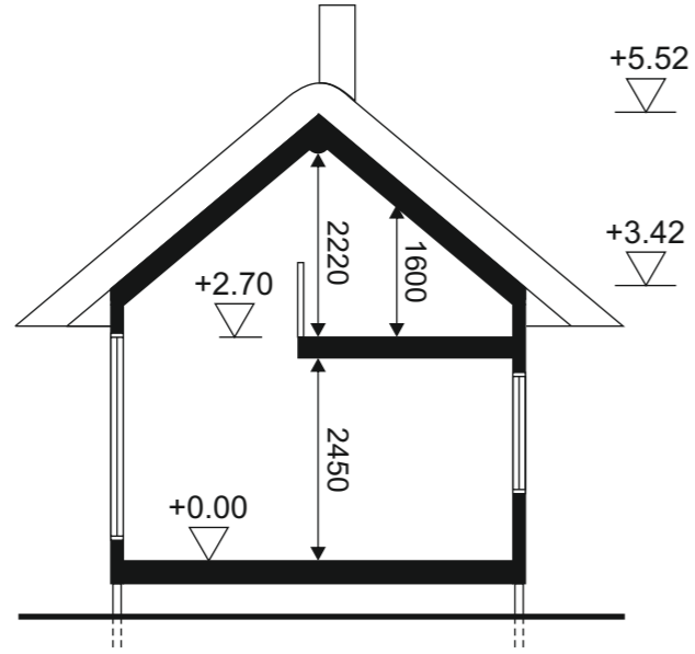
LEIKKAUS
