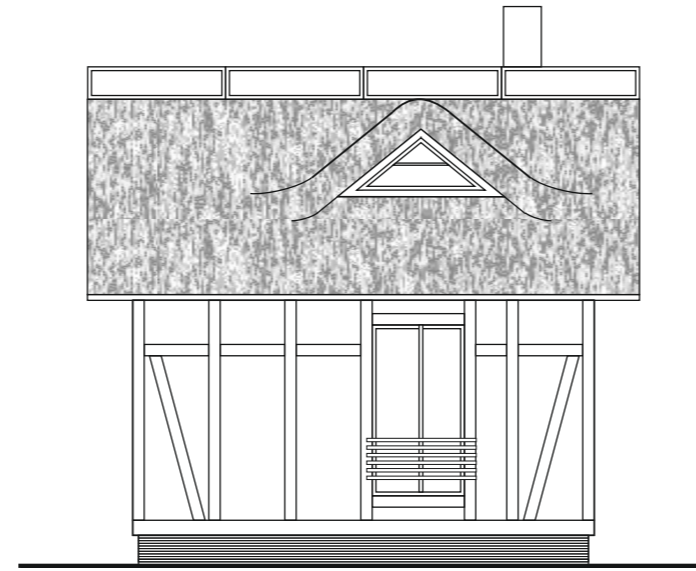
TAKAJULKISIVU
