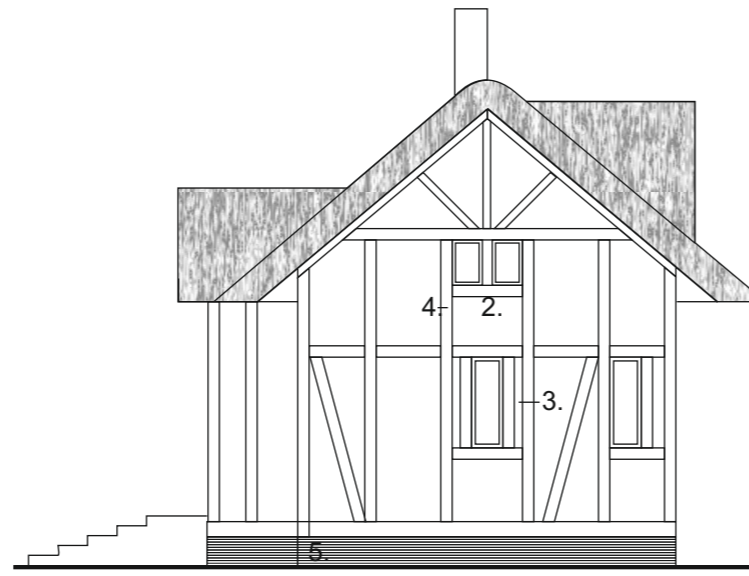
PÄÄTY
