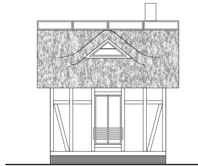
PÄÄTY
