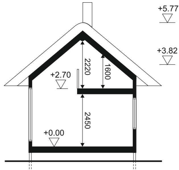
LEIKKAUS
