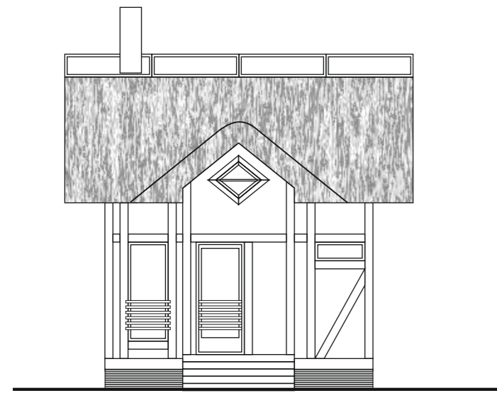
SISÄÄNKÄYNTIJULKISIVU
