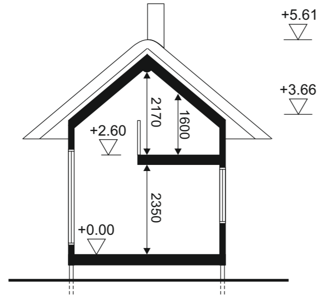
LEIKKAUS
