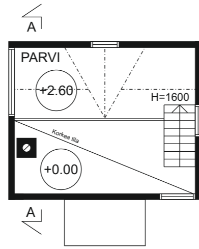
POHJA-PIIRUSTUS PARVI
